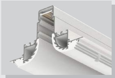
KLM-GD13075Y/H Cut hole: W90*H85mm
